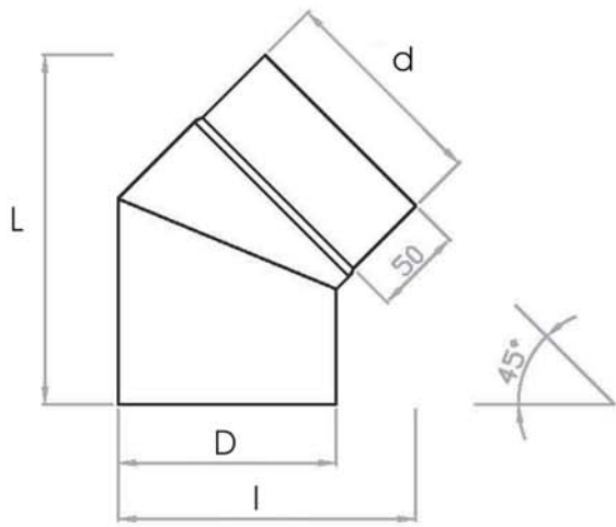
Koleno 45°
