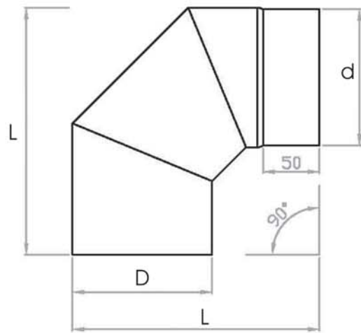
Koleno 90°
